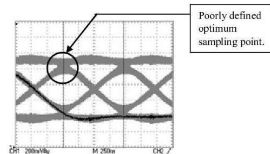
그림 12-4. 왜곡된 눈(eye) 다이어그램
