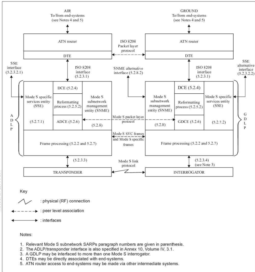
모드 S 서브 네트워크의 기능적 요소들
