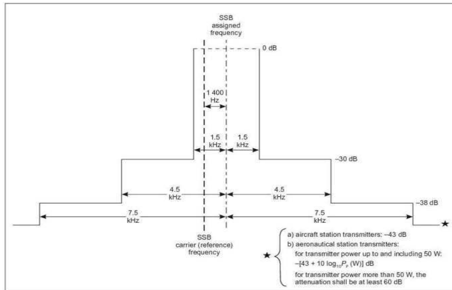
그림 2-2. 1983. 2. 1 이후 최초 설치된 항공국 송신기와 1983년 2월 1일 이후 사용 중인 항공국 송신기에 필요한 스펙트럼 한계(피크 파워 기준)
