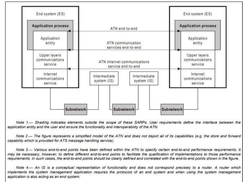
그림 3-1. ATN의 개념적 모델
