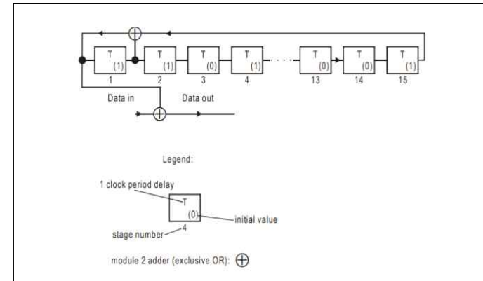
그림 6-2. 비트스크램블링 시퀀스에 대한 PN-발생기
