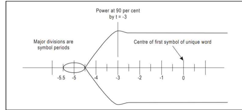
그림 6-1. 송신기 전력 안정화
