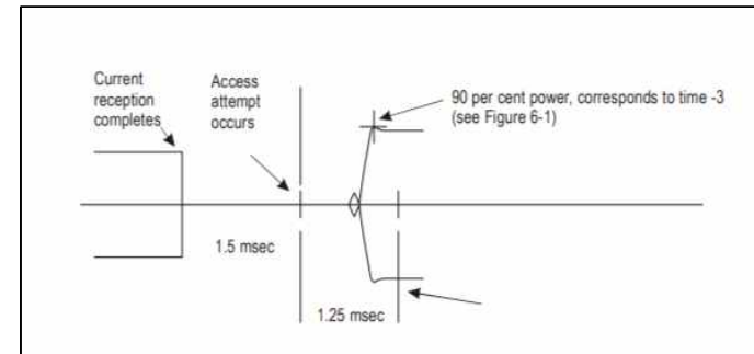
그림 6-3. 수신에서 송신으로의 전환 시간
