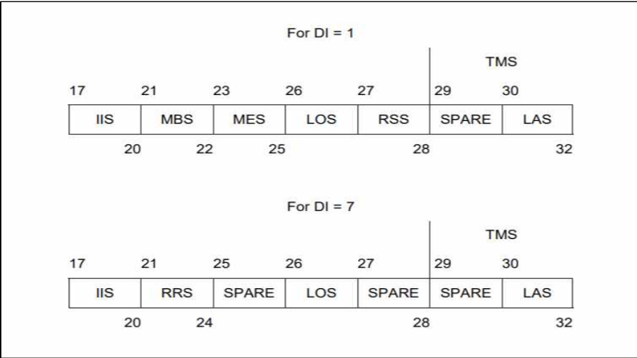
그림 5-1. SD 필드 구조
