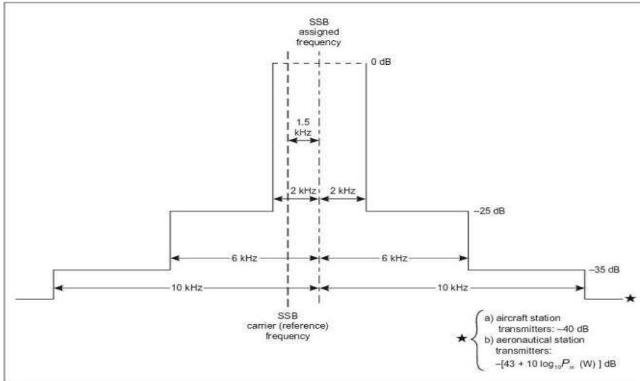
그림 2-1. 1983. 2. 1 이전에 처음 설치된 항공국 송신기와 항공국 송신기에 필요한 스펙트럼 한계(평균 파워 기준)
