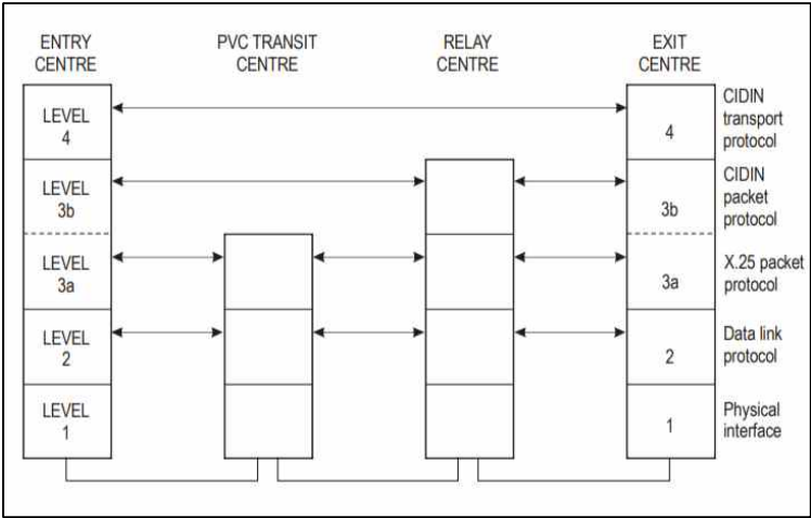
그림 8-1. CIDIN 통신프로토콜 레벨
