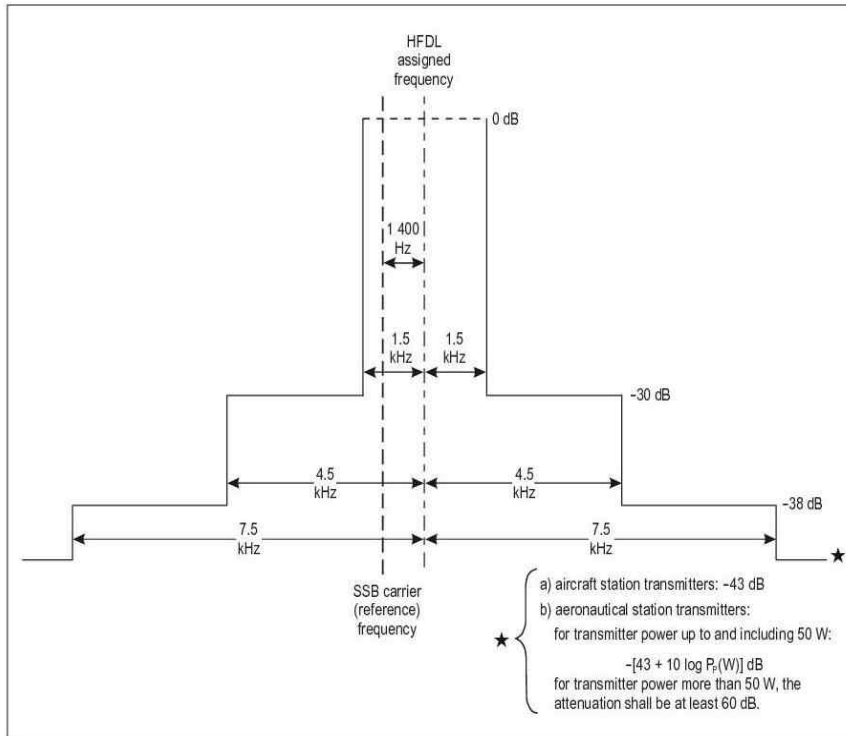
그림 11-1. HF DL 항공기와 지상국 송신기에 대한 침투전력에 대한 요구 스펙트럼 제한
